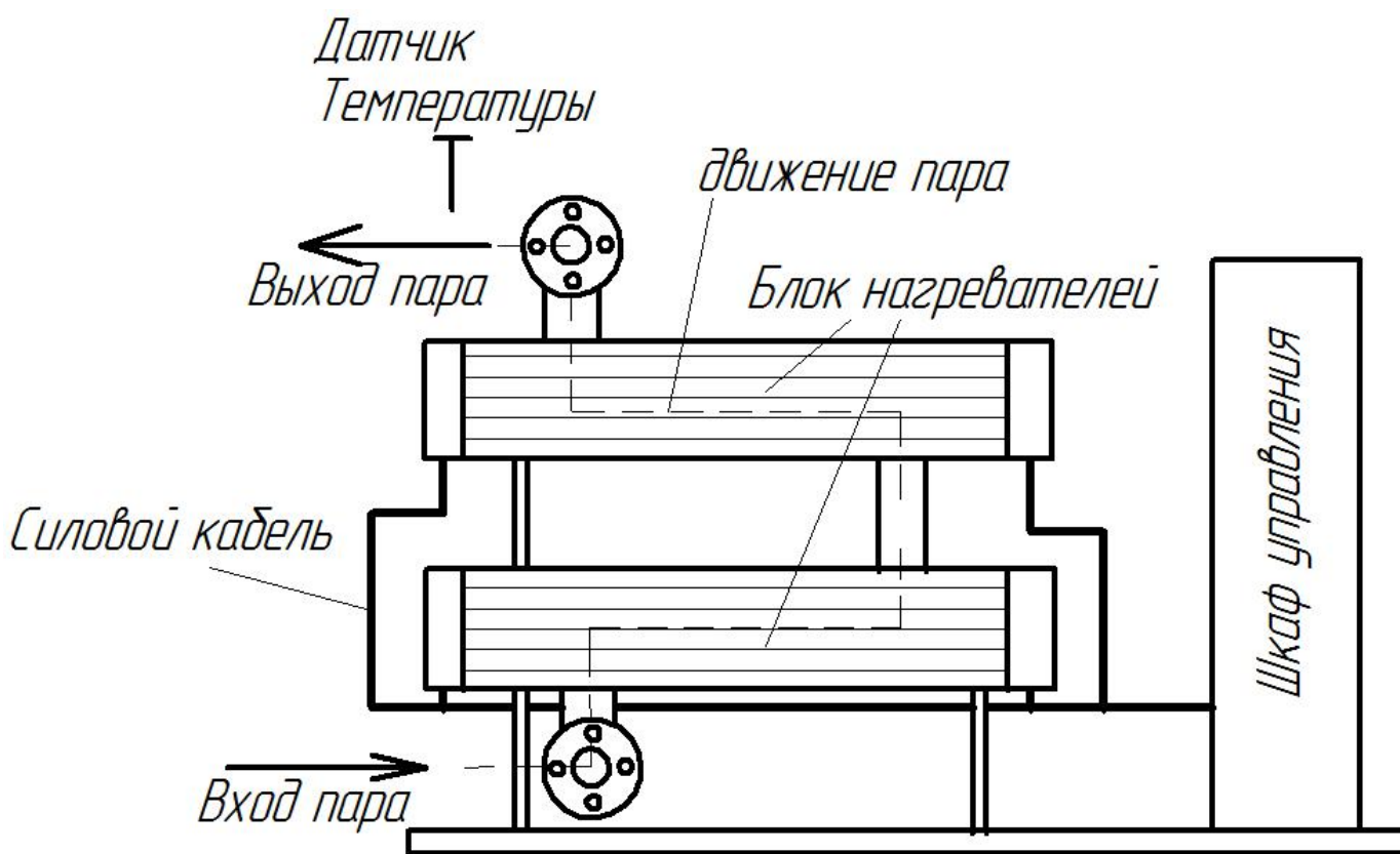
Общая схема пароперегревателя ПП
